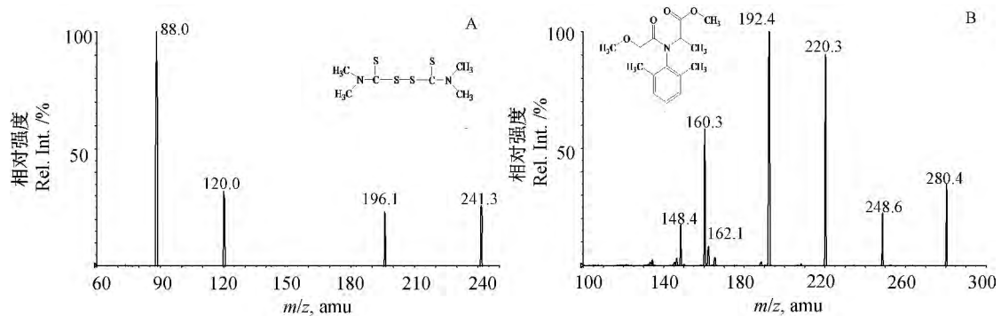
图1 福美双(A)和甲霜灵(B)二级质谱图
