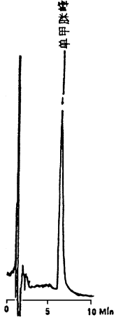
图 1 单甲脒标准溶液的 HPLC 图
