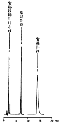
图 2 2,4-二甲氨基苯胺、单甲脒、双甲脒的混标 HPLC 图
