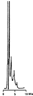
图 5 柑桔空白试样的 HPLC 图
