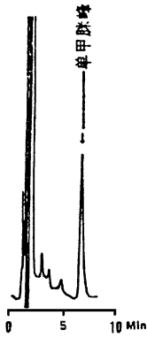
图 4 苹果加标试样的 HPLC 图
